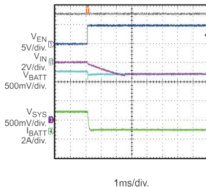
En Off
