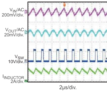
Input/Output Ripple
