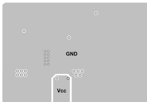
Inner Layer1
