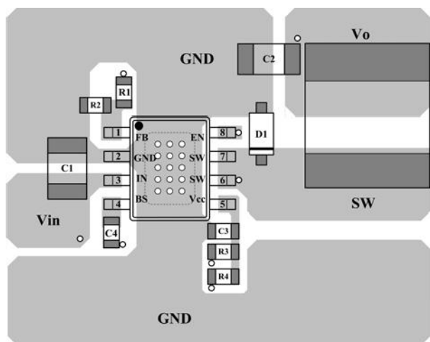
Top Layer
