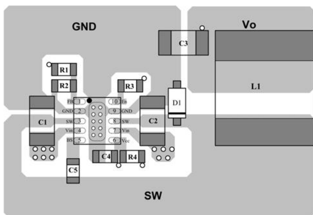
Top Layer
