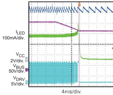
V_{BUS} Turn Off
