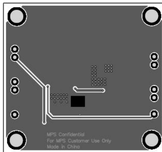
Figure 6—Bottom Layer
