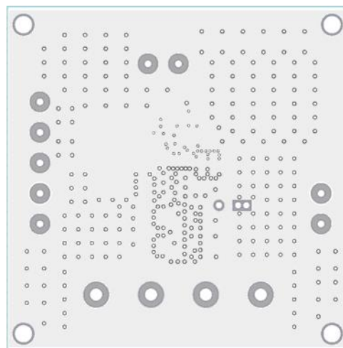
Inner2 Layer
