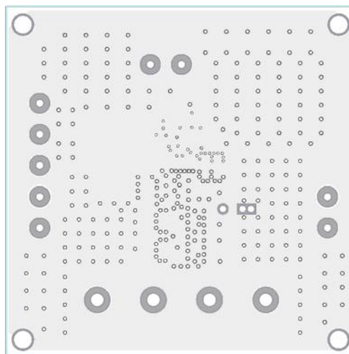
Inner1 Layer
