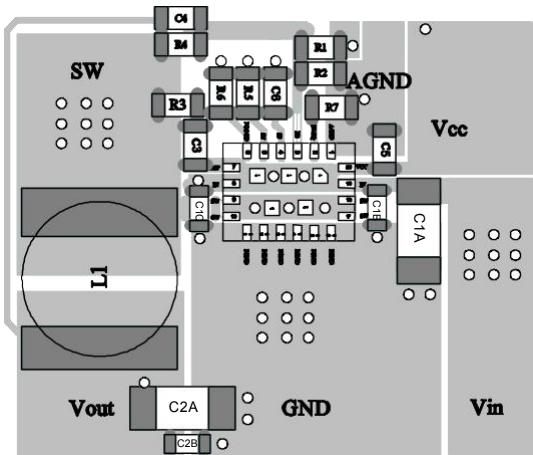
Top Layer
