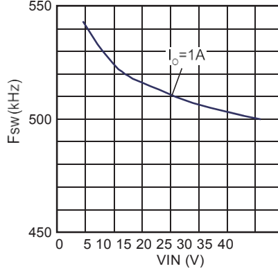
Fsw vs. VIN
