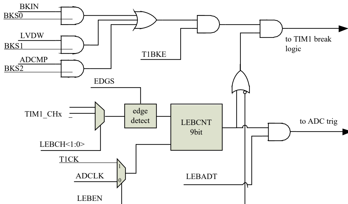
图 10.40 前沿消隐原理框图
