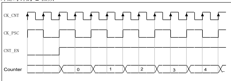
图 10.16 内部时钟源并且预频为 1 时，计数器计数时序图
