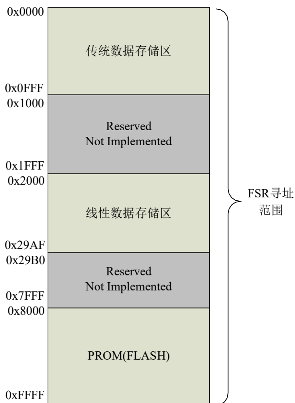
图 3.4 间接寻址
