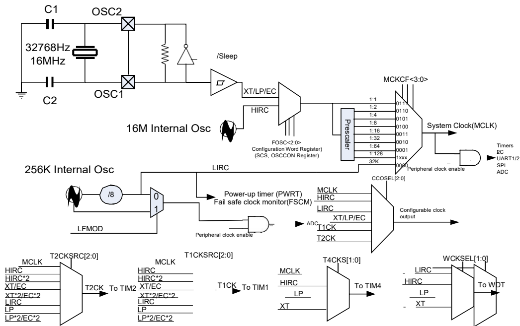
5.1 系统时钟源框图
