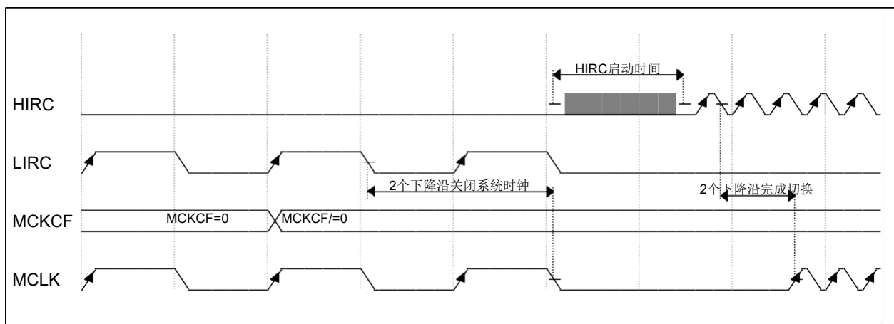
图 5.2 由慢时钟切换到快时钟
