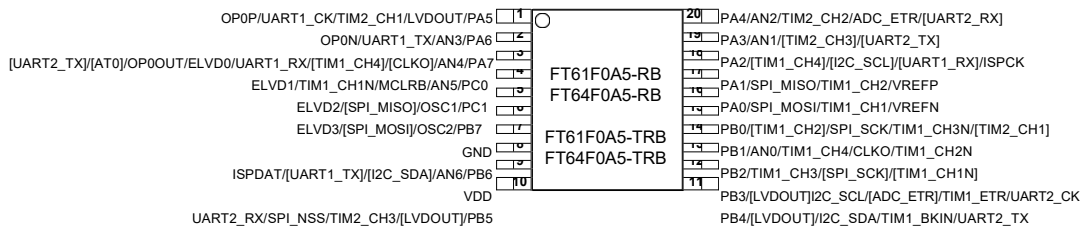
图 1.5 SOP20, TSSOP20 脚位
