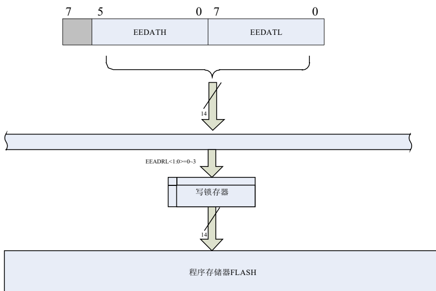
图 8.3.2 对带 1 个写锁存器的 FLASH 进行写操作
