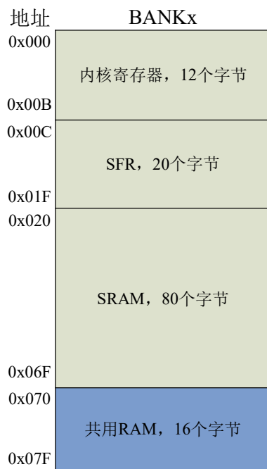
图 3.1 存储区构成
