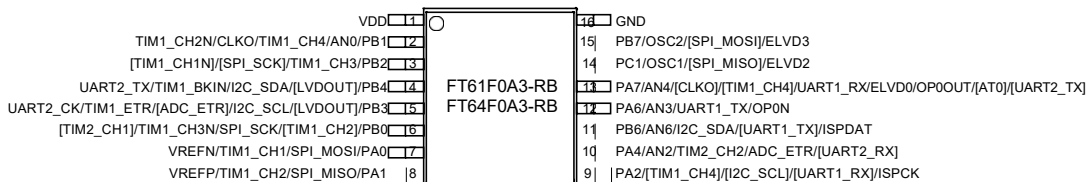
图 1.4 SOP16 脚位
