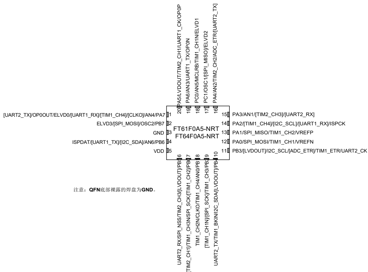
图 1.6 QFN20 脚位
