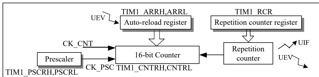
图 10.2 计数基本单元
