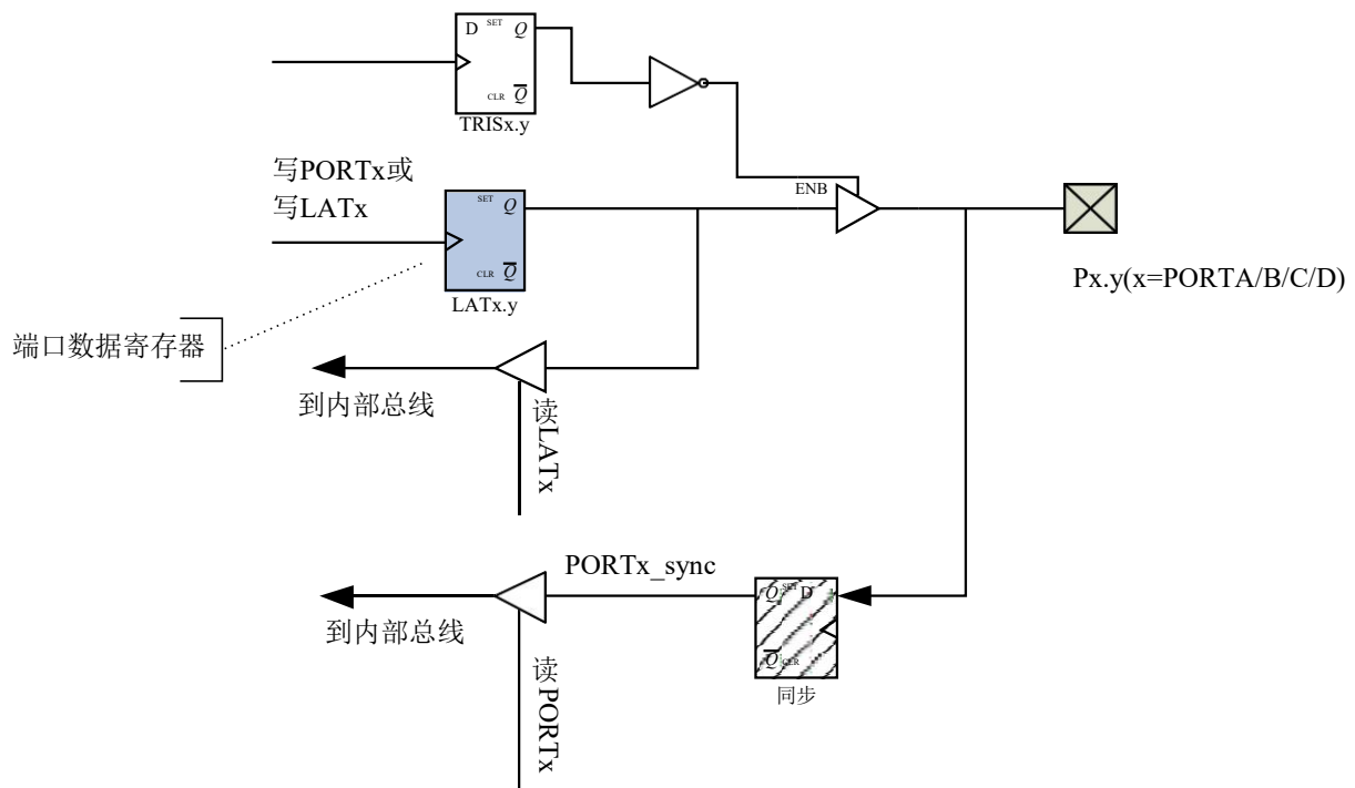
图 16.3 端口读操作原理框图
