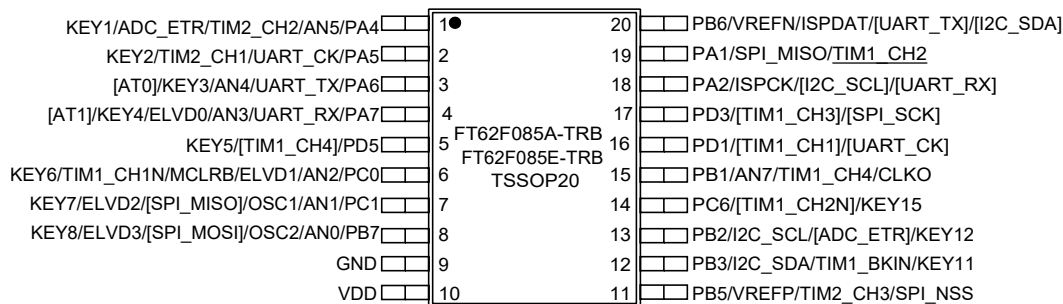
图 1.2 TSSOP20 脚位
