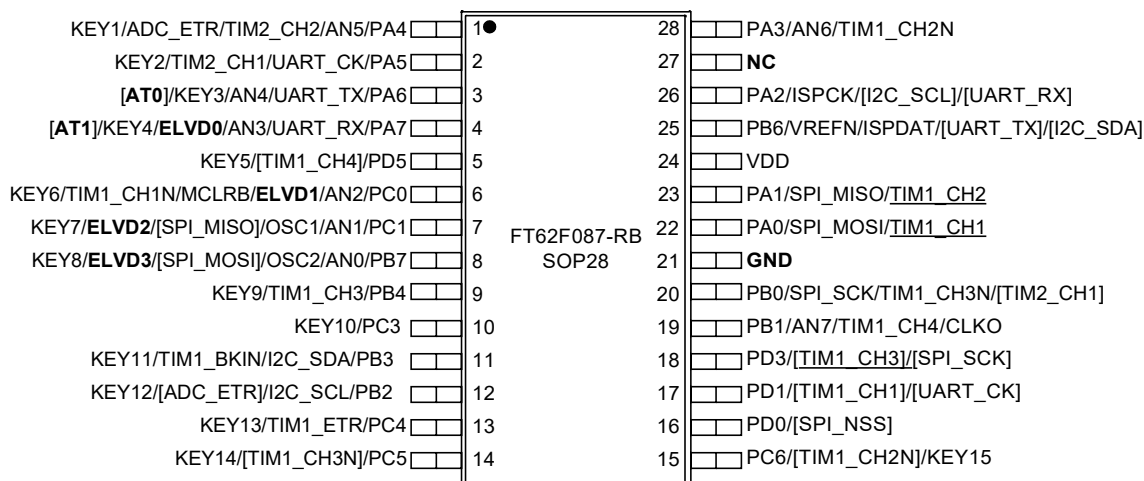
图 1.5 SOP28 脚位
