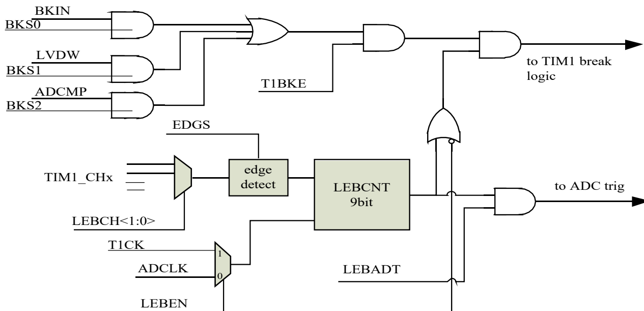
图 10.36 前沿消隐原理框图
