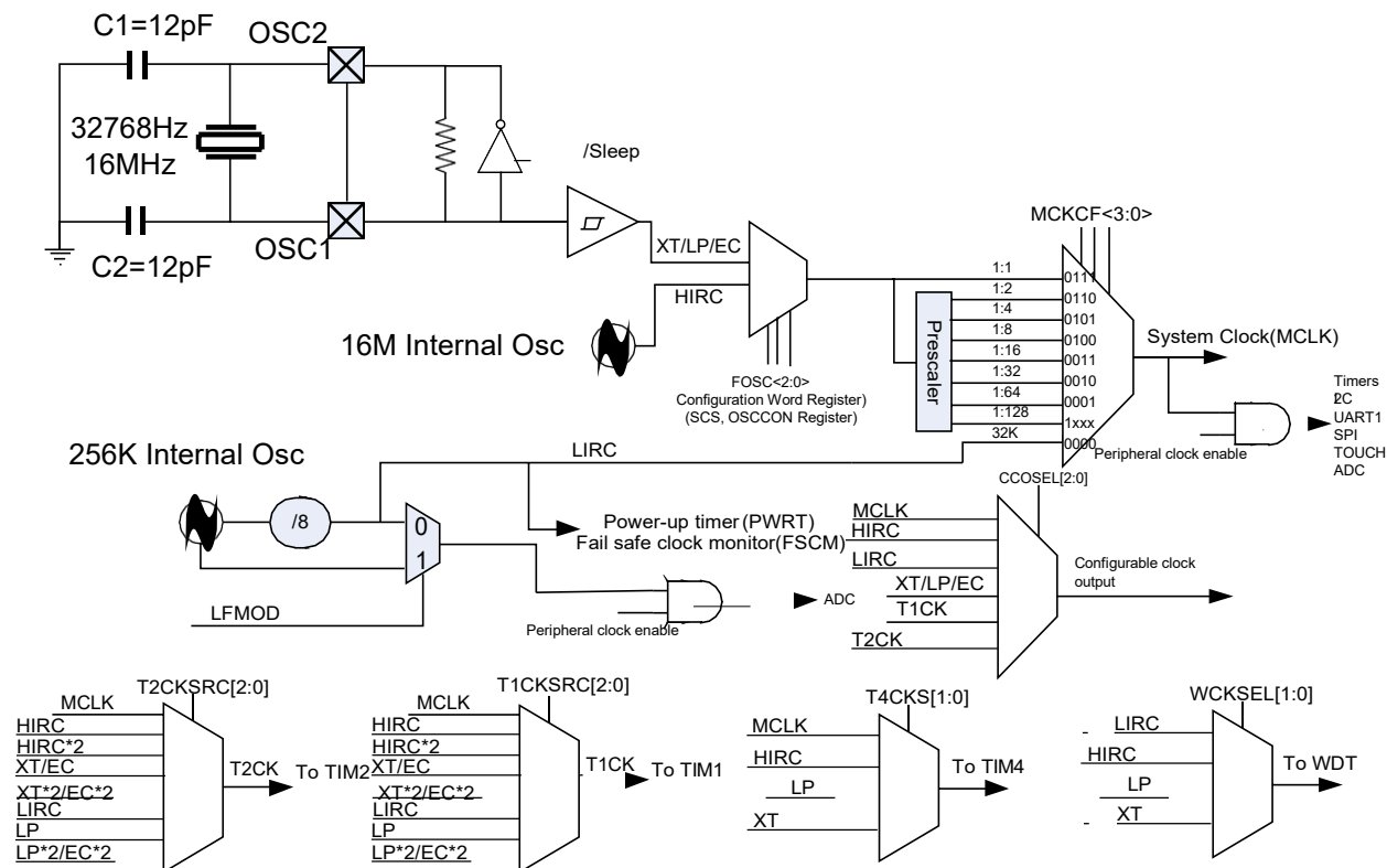
5.1 系统时钟源框图
