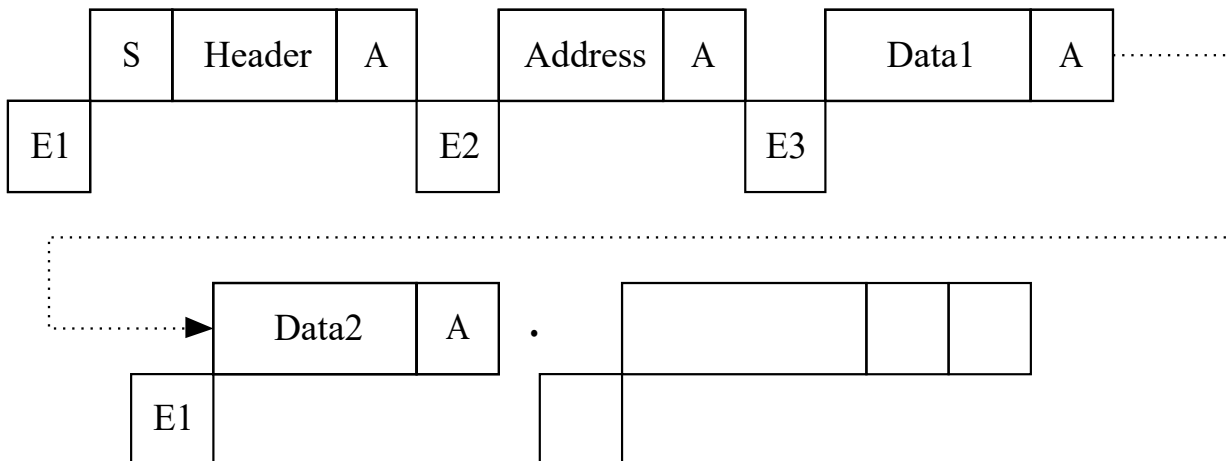
图 14.3 10 比特地址模式主机发送流程图
