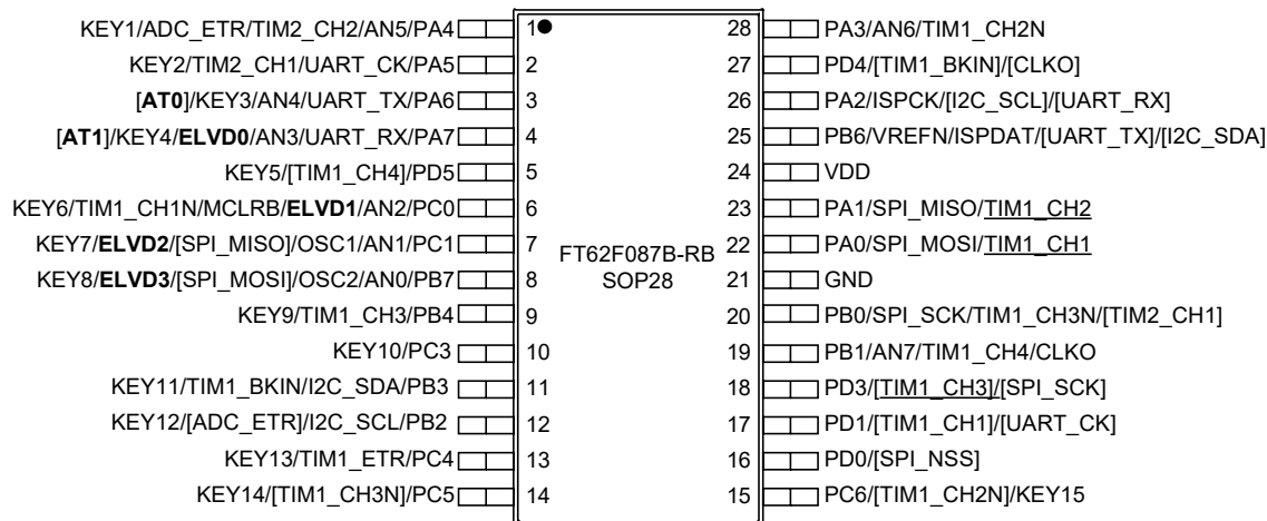
图 1.7 SOP28 脚位 B
