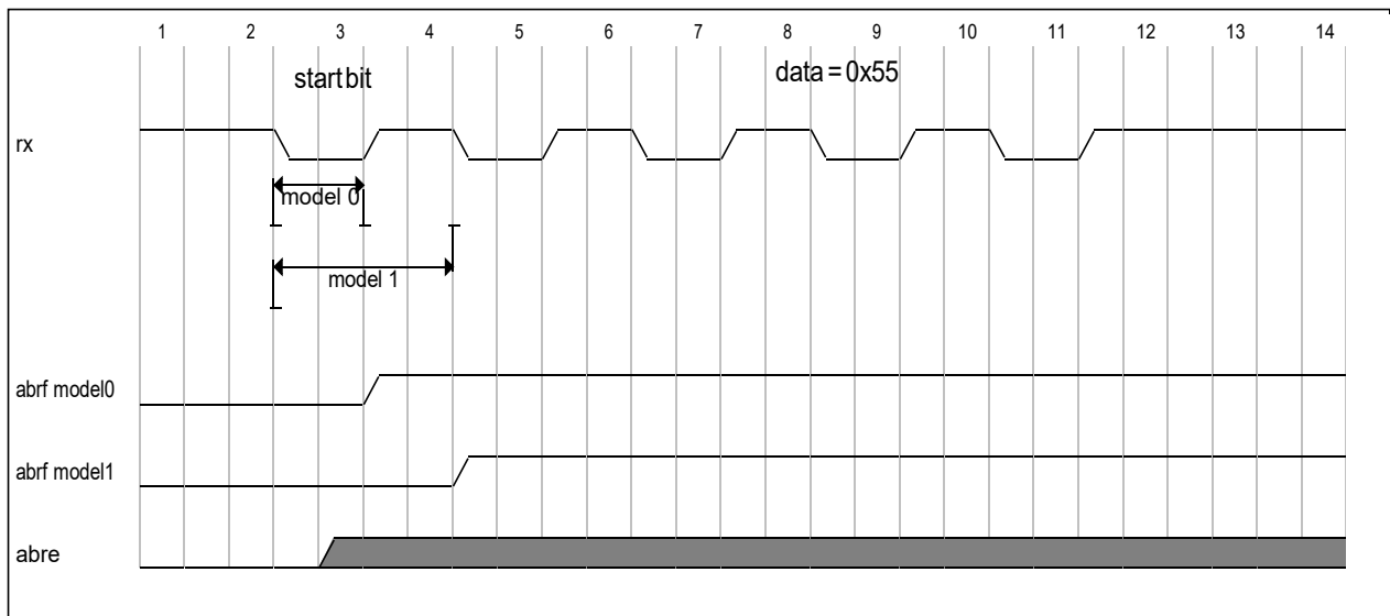
图 15.11 自动波特率检测时序图
