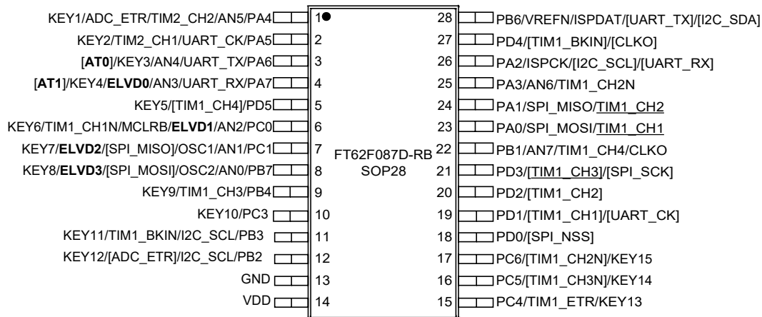
图 1.9 SOP28 脚位 D
