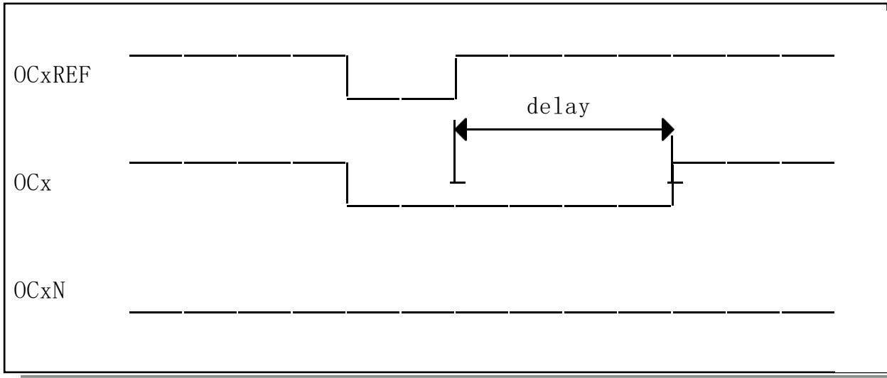
图 10.32 正向输出被死区覆盖时序图
