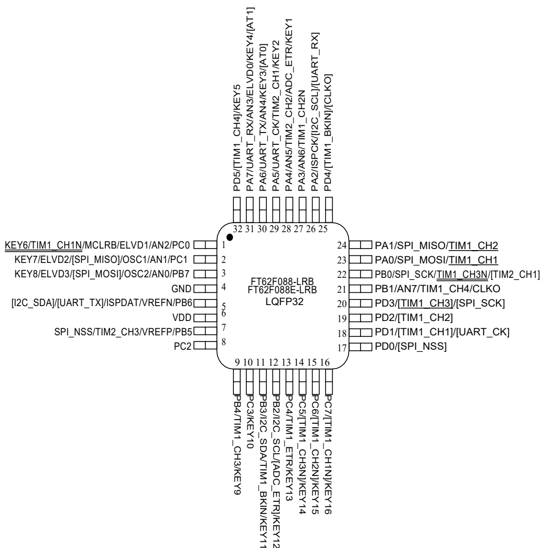
图 1.6 LQFP32 脚位
