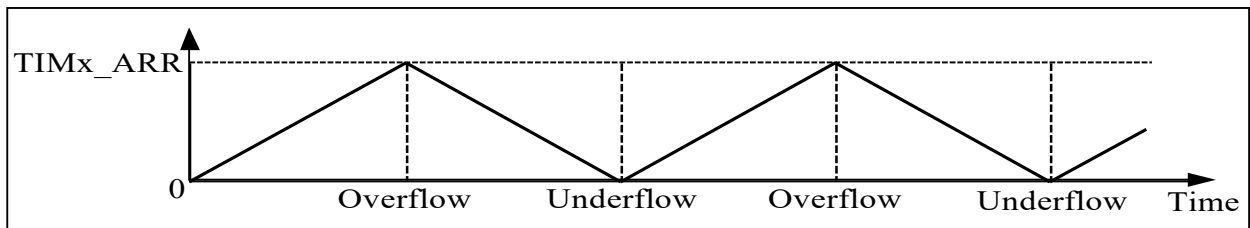
图 10.11 中心对齐模式，T1DIR 初始化为 0
