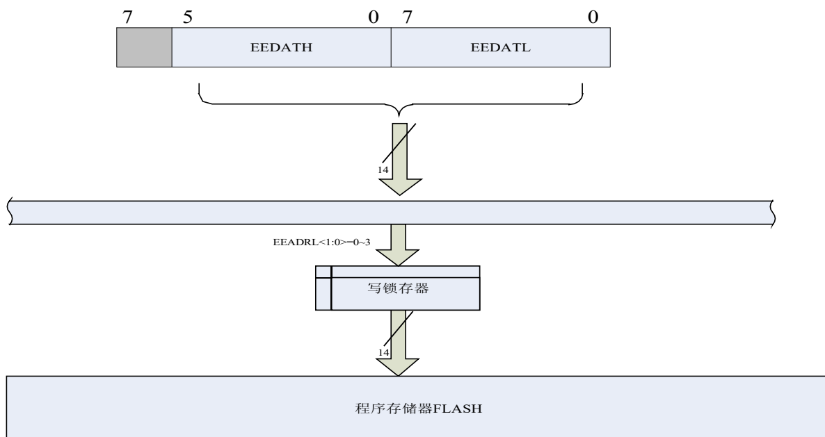
图 8.3.2 对带 1 个写锁存器的 FLASH 进行写操作
