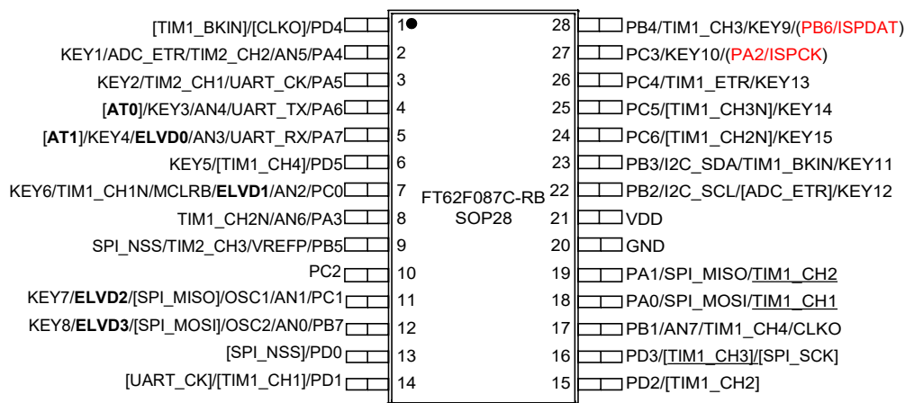
图 1.8 SOP28 脚位 C
