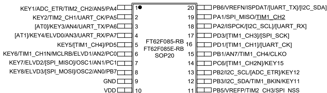
图 1.3 SOP20 脚位
