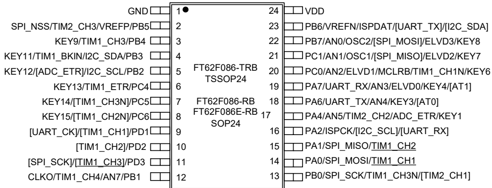
图 1.4 SOP24/TSSOP24 脚位
