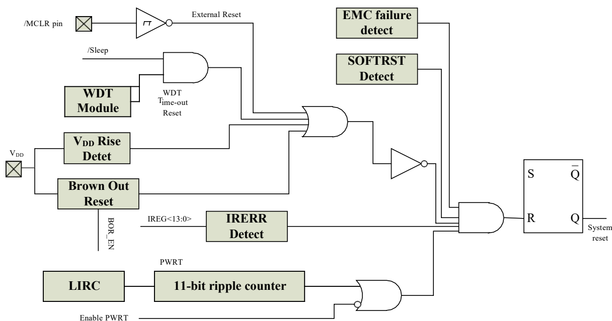
图 4.1 复位框图
