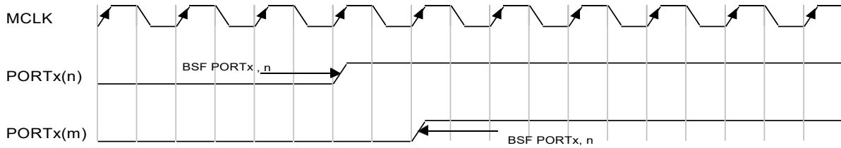
图 17.4 连续使用 RMW 指令对 PORTx 写操作的期望时序
