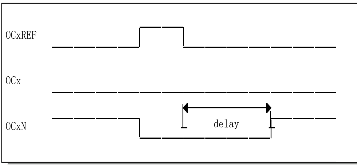
图 10.32 正向输出被死区覆盖时序图
