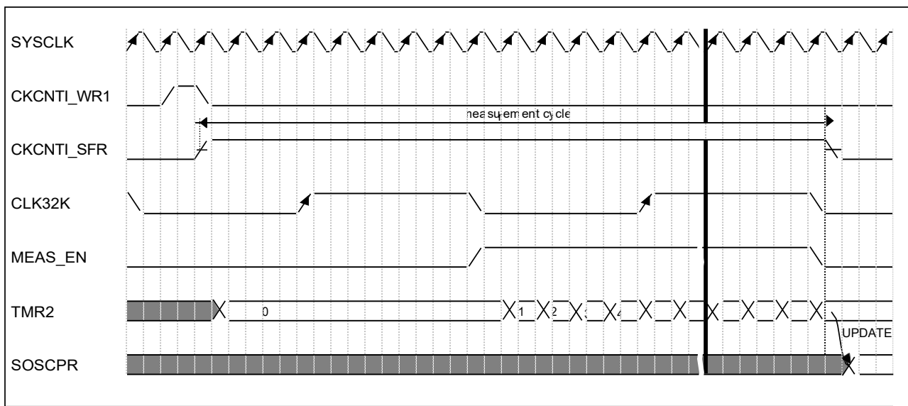
图 15.2 单次测量时序示意图（CLK32K 和 SYSCCLK 未按真实比例画）
