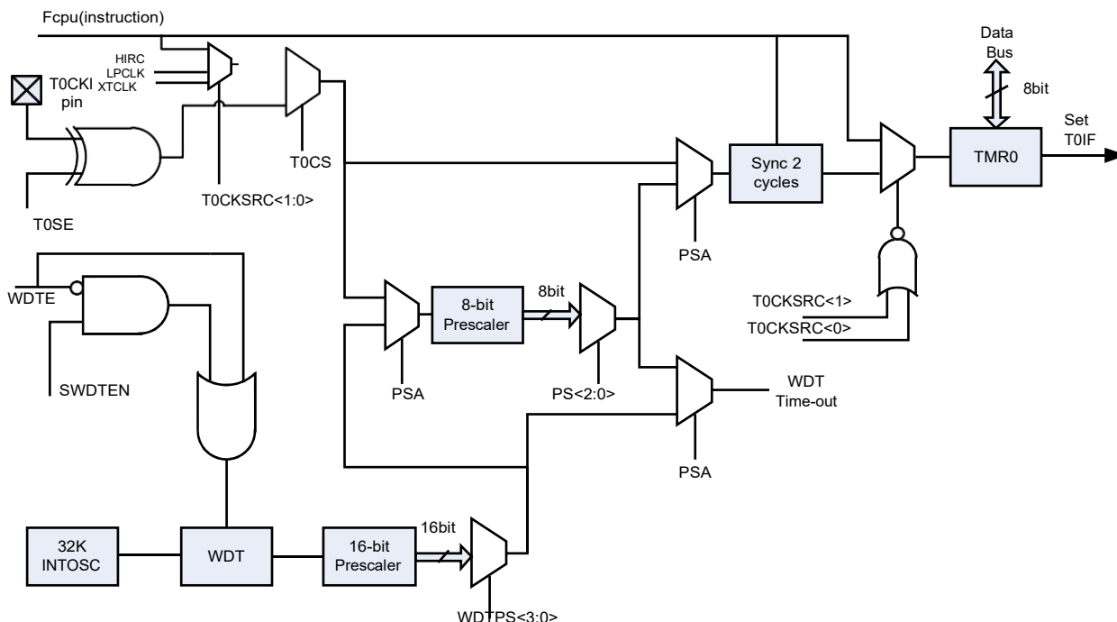
图 10.1 看门狗和定时器 0 框图
