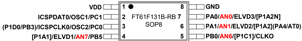
图 1.2 SOP8 脚位
