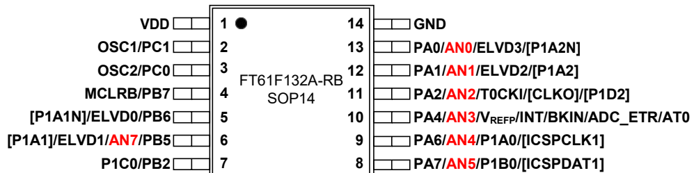
图 1.4 SOP14 脚位
