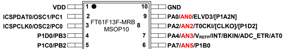
图 1.3 MSOP10 脚位
