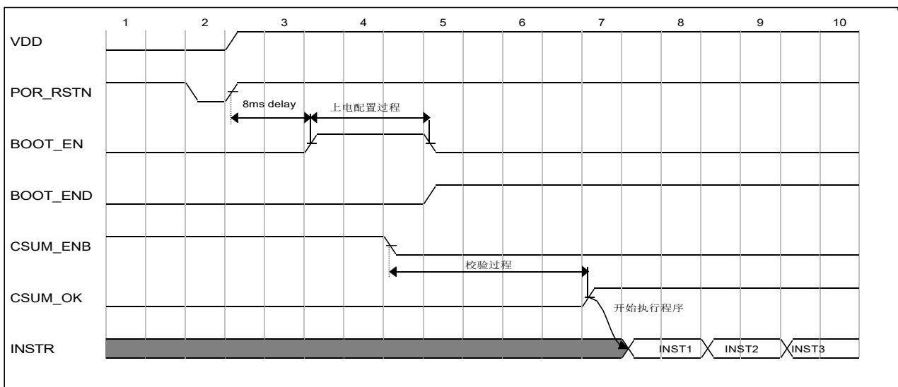
图 4.5 校验过程
