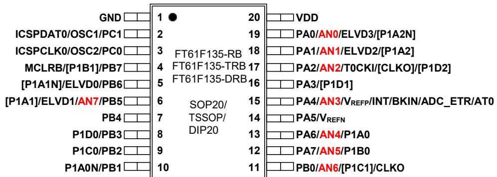
图 1.6 SOP20/TSSOP20/DIP20 脚位
