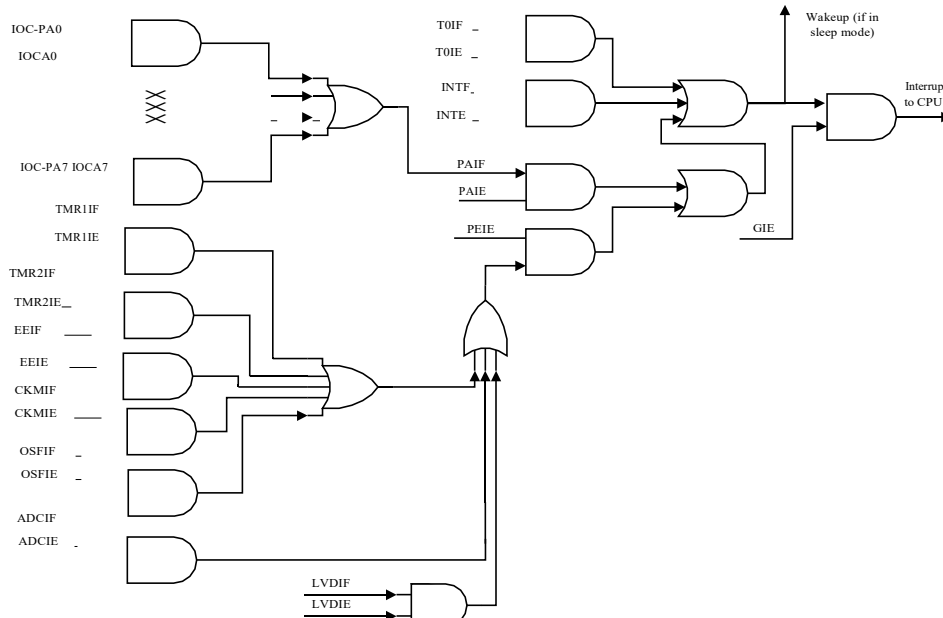
图 6.1 中断逻辑框图
