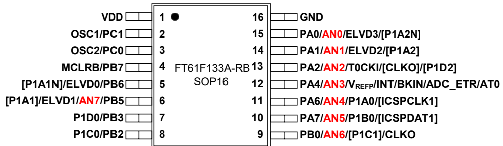
图 1.5 SOP16 脚位
