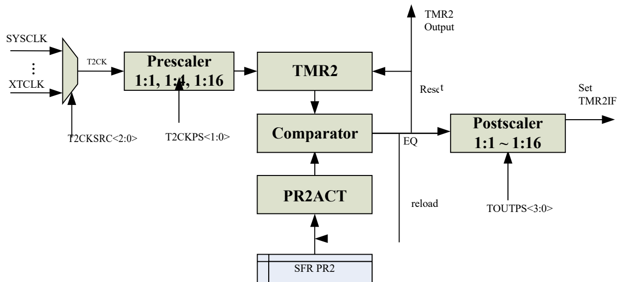
图 7.1 定时器 2 框图
