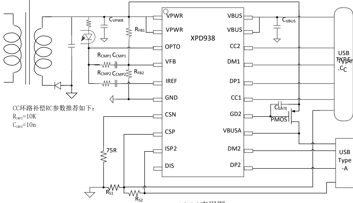
AC-DC应用图
