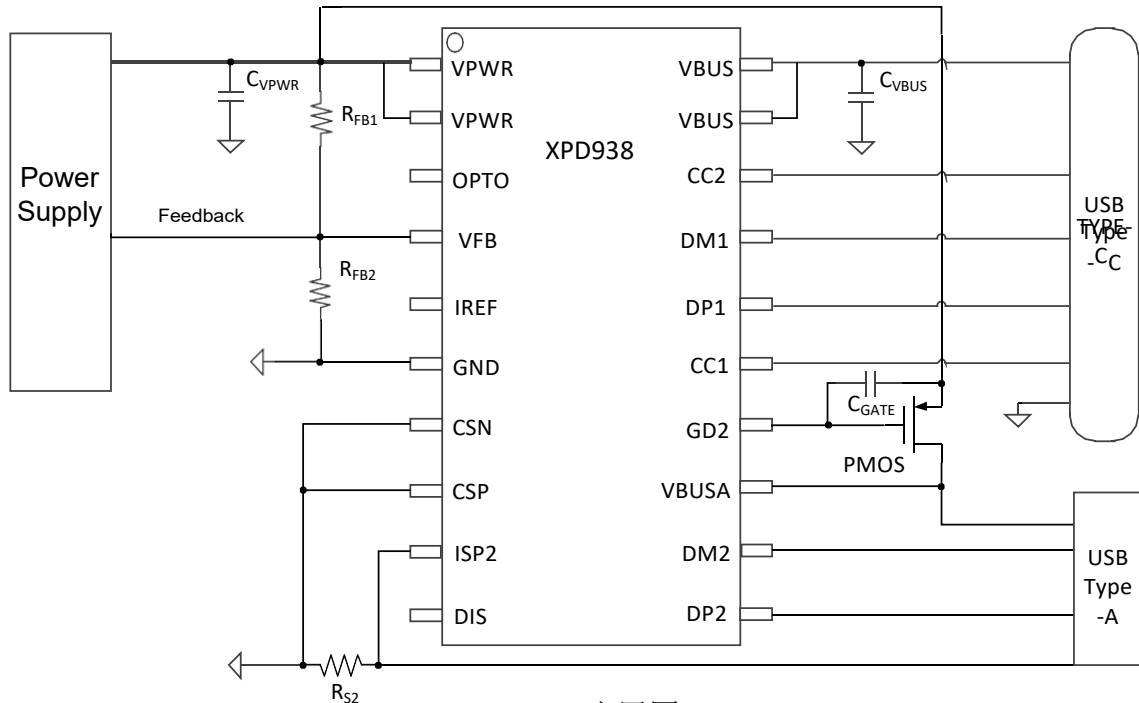
DC-DC应用图
