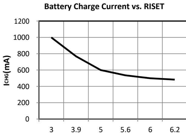
Figure2 R_{ISET} (kΩ)
