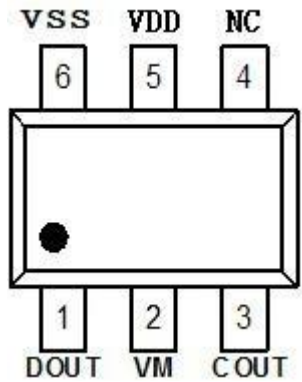
SOT23-6
