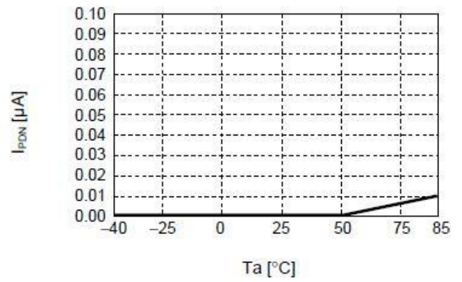
4. I_{PDN}-T_a
