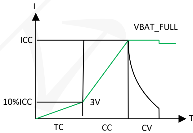
图(3) XPM6320 充电过程示意图
