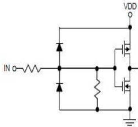
LE 输入端
